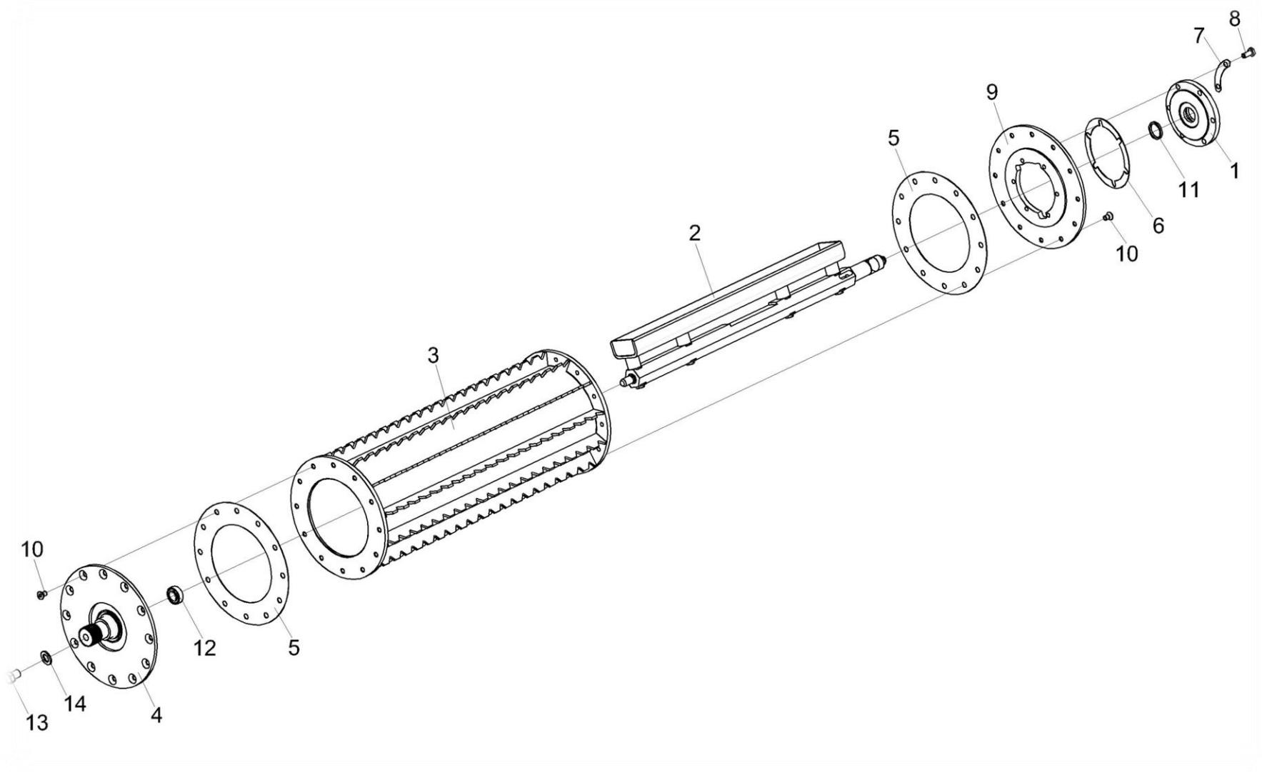
Рисунок 66 – Валец нижний передний КВС-8-0111210Б
