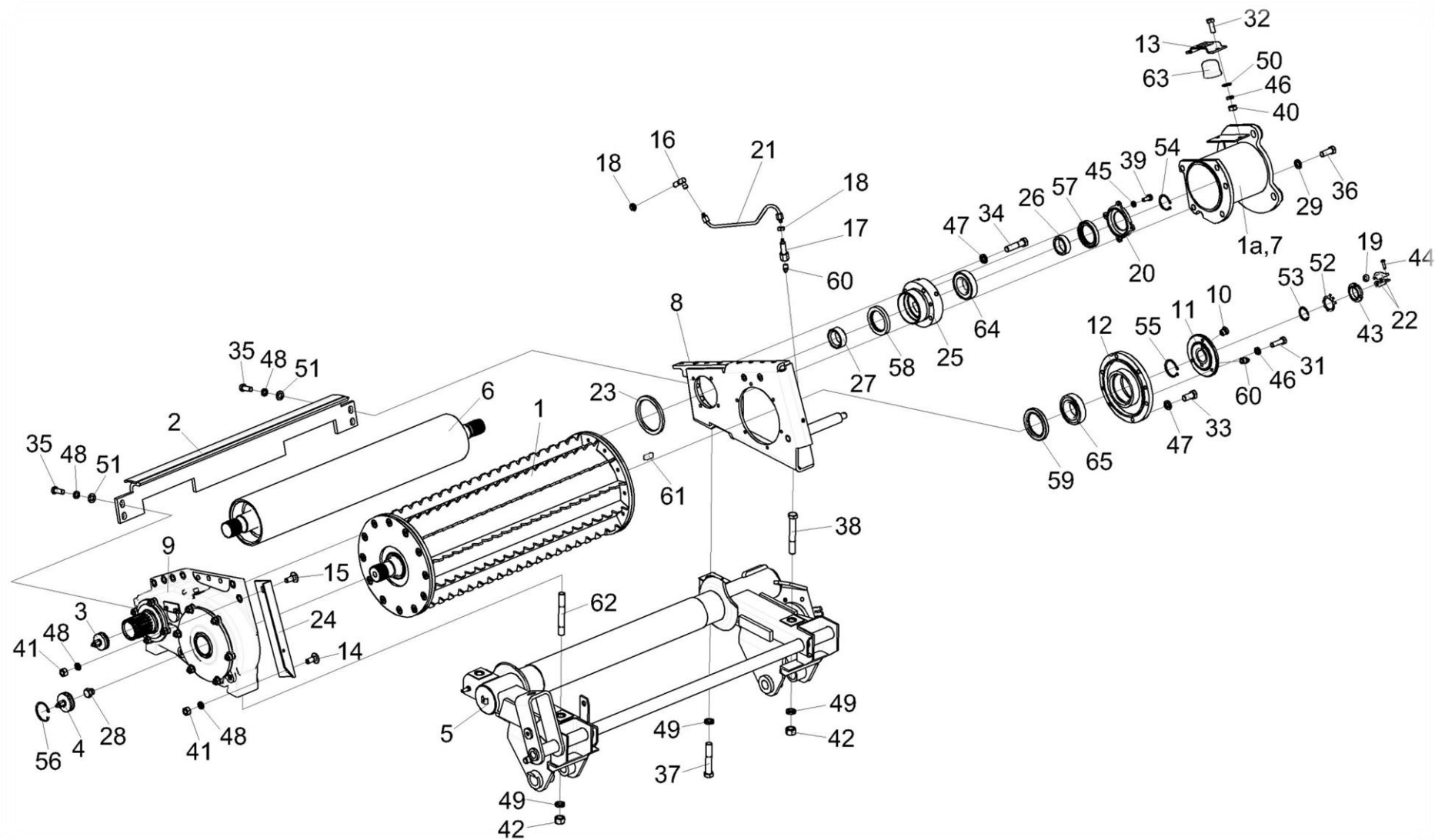
Рисунок 65 – Вальцы нижние КВС-8-0111200Б
